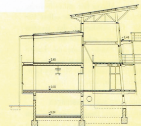
Systemquerschnitt M 1:175
